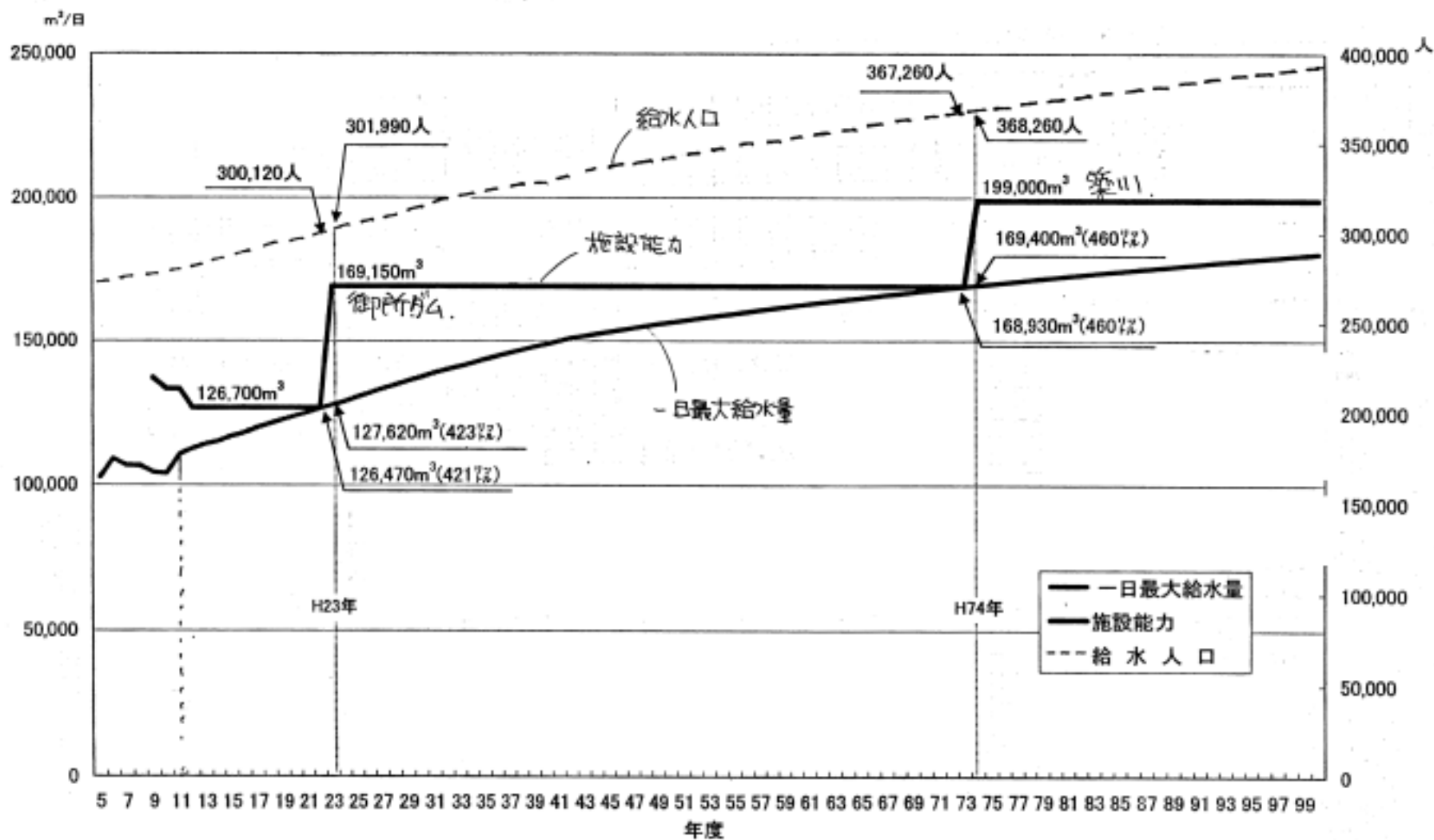
図2 盛岡市の計画給水量と施設能力
